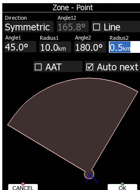
Wendepunktsektor in Form des bei Wettbewerben gebräuchlichen „Schlüsseloches“
